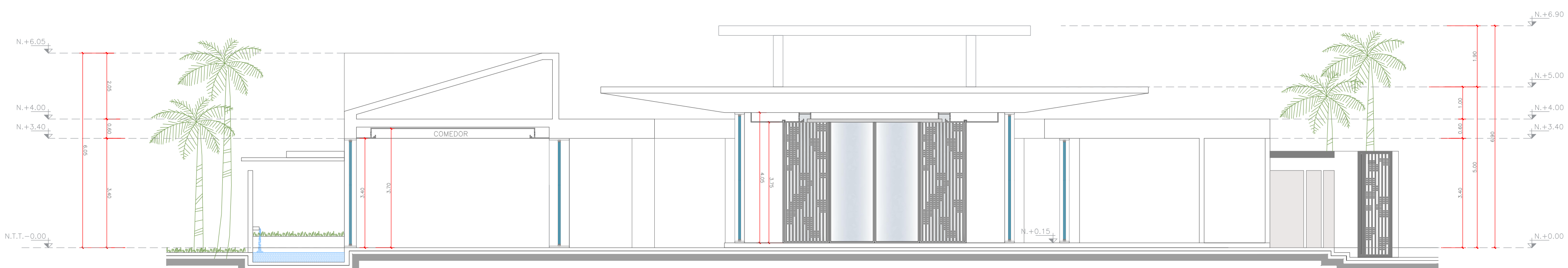
SECCION D-D
